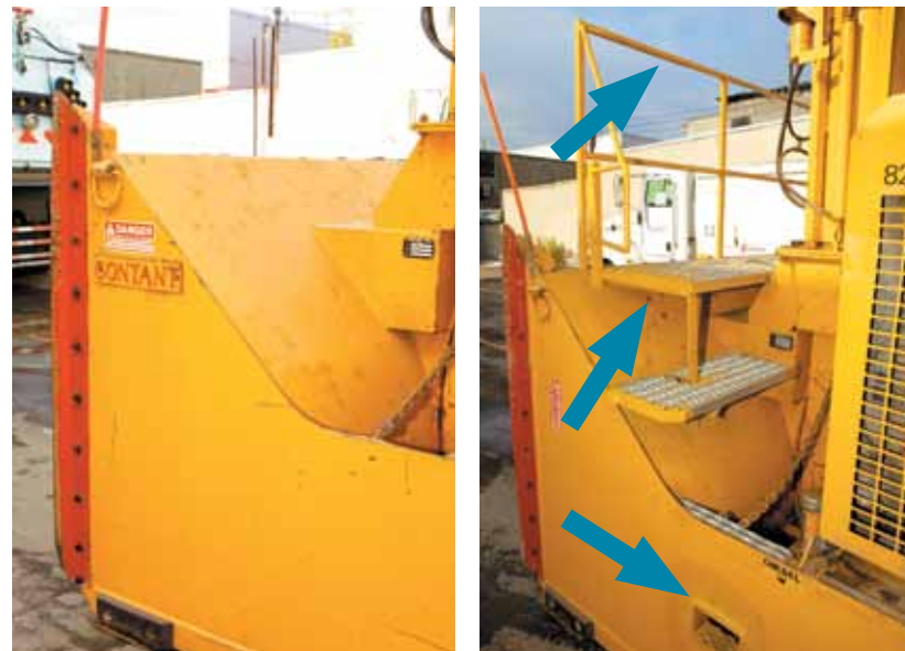
La souffleuse avant (à gauche) et après (à droite) les améliorations.
