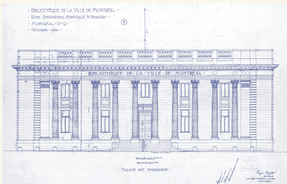
Plan de construction de la Bibliothèque de la Ville de Montréal : façade, rue Sherbrooke. Par Eugène Payette, architecte. 1914. VM116-1_0039-B-1029-001. Archives de la Ville de Montréal.
