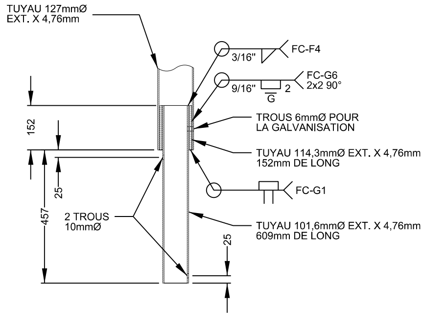
COUPE A-A
