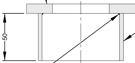
COUPE A-A
