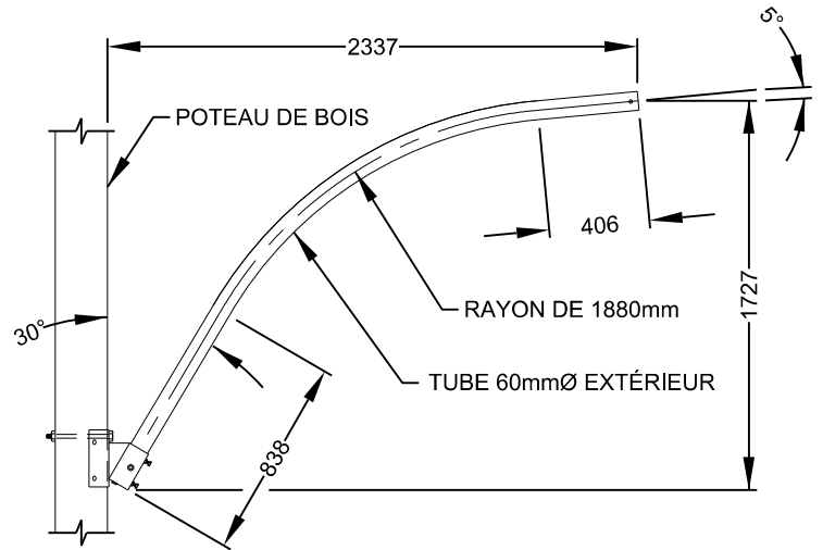
ÉLÉVATION
