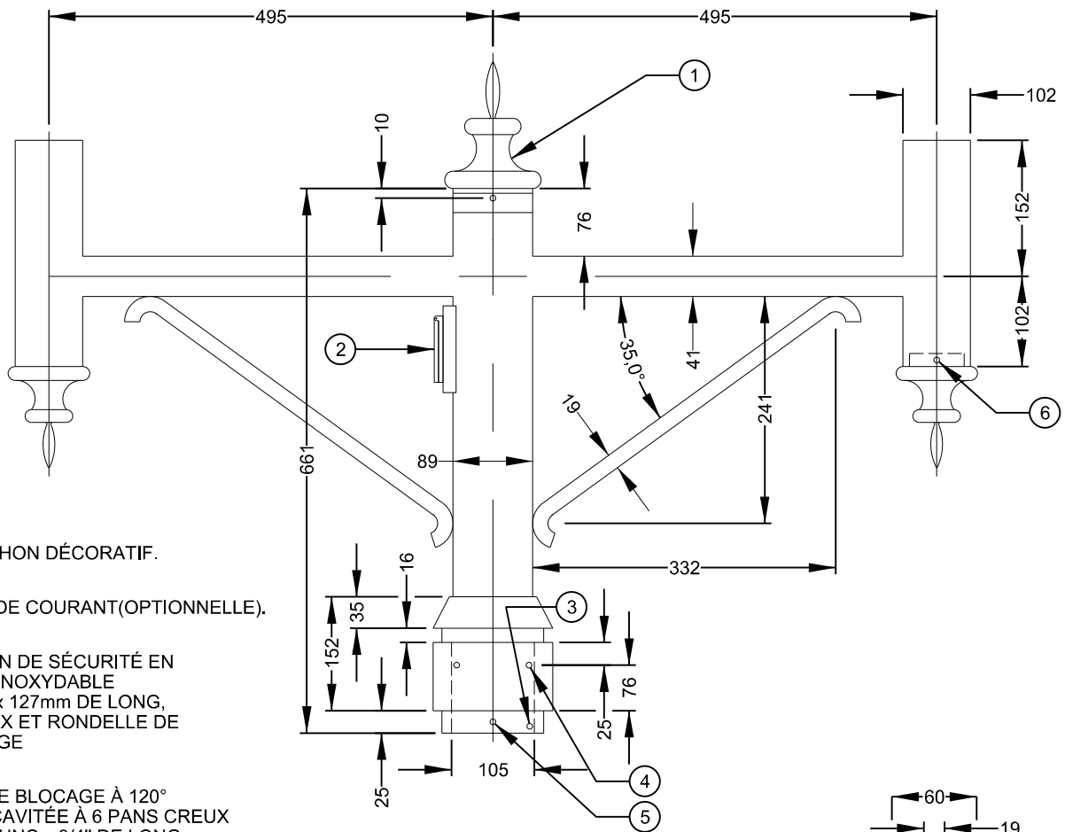
ÉLÉVATION
