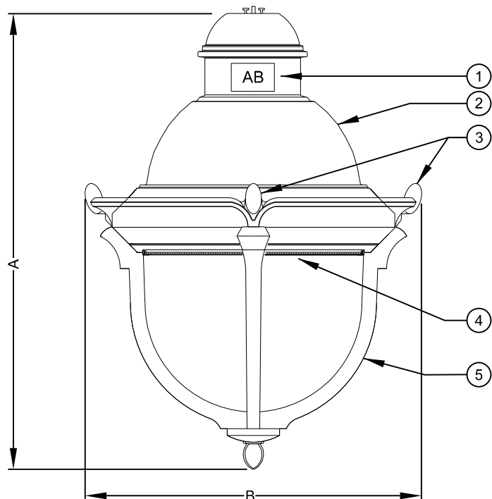
ÉLÉVATION
