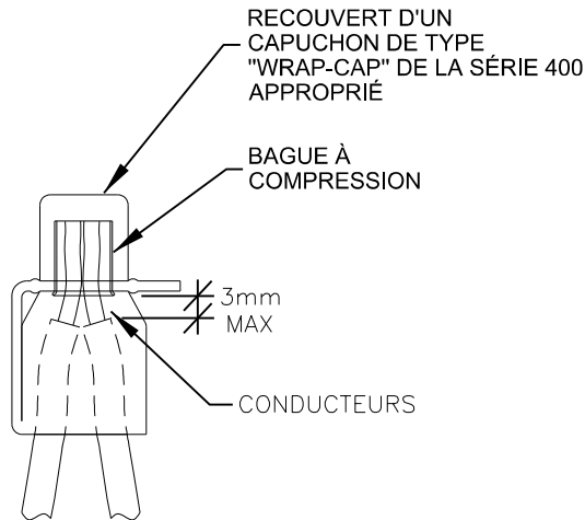
FIGURE 1 BAGUE À COMPRESSION AVEC CODE DE COULEUR
