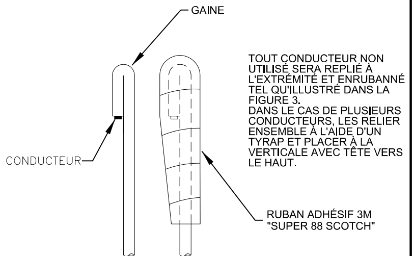
FIGURE 3 CONDUCTEURS NON UTILISÉS
