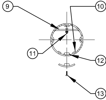
COUPE A-A
