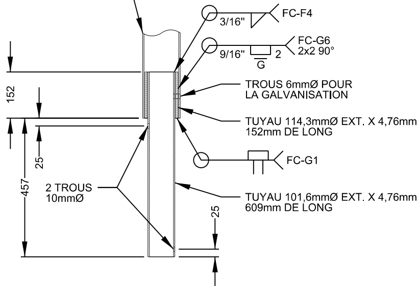
COUPE A-A
