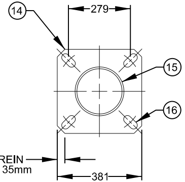
SEMELLE D'ANCRAGE
