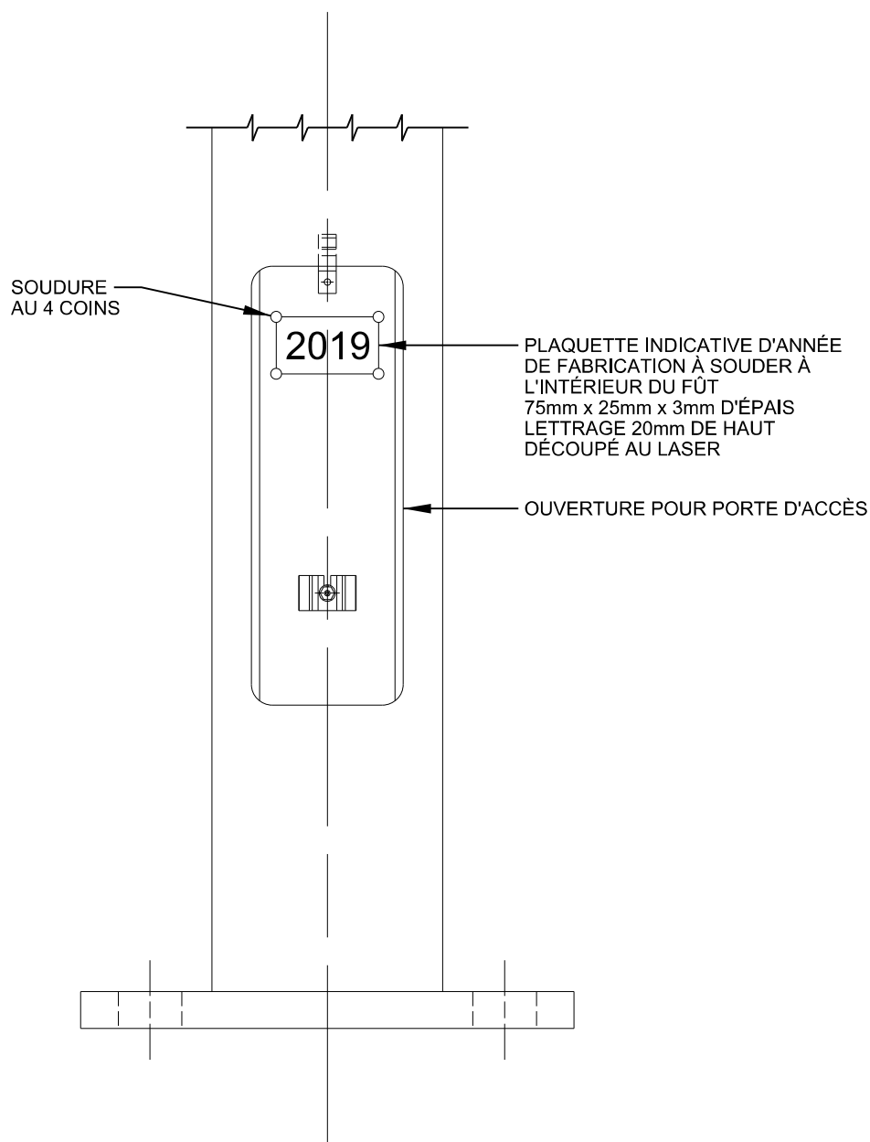
ÉLÉVATION
