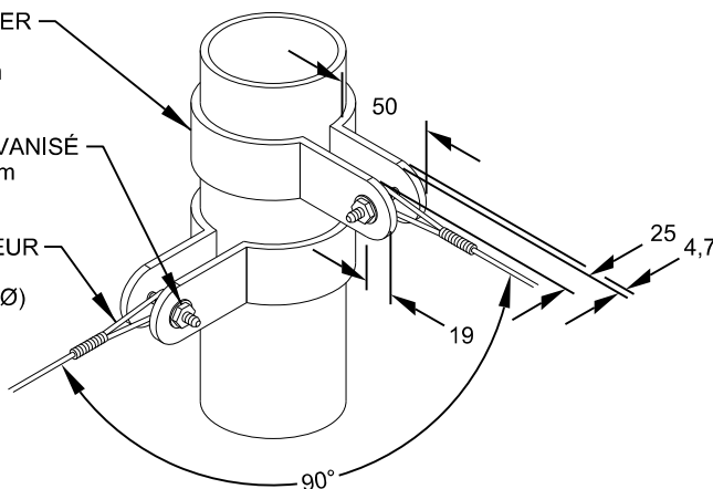
DÉTAIL BRIDE DE FIXATION
