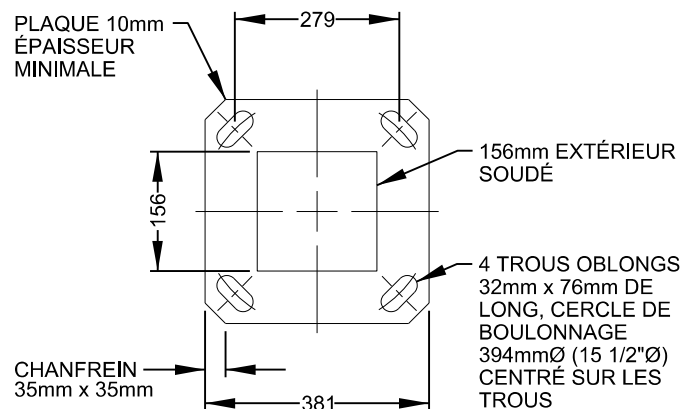
SEMELLE D'ANCRAGE
