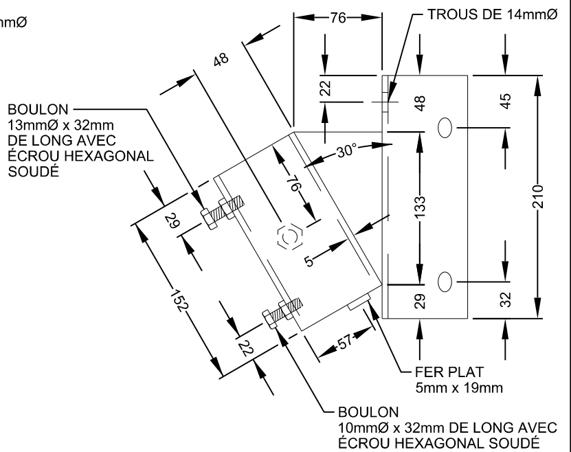
DÉTAIL DE L'APPLIQUE
