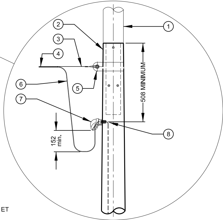
DÉTAIL "A"
