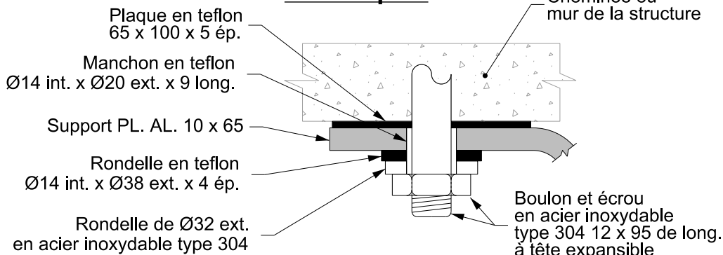
Détail A
