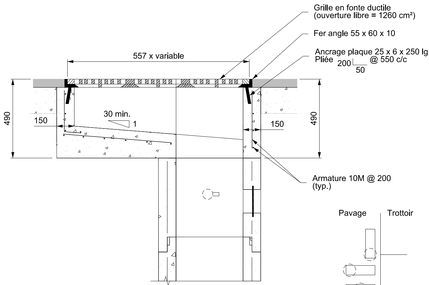
Coupe A-A
