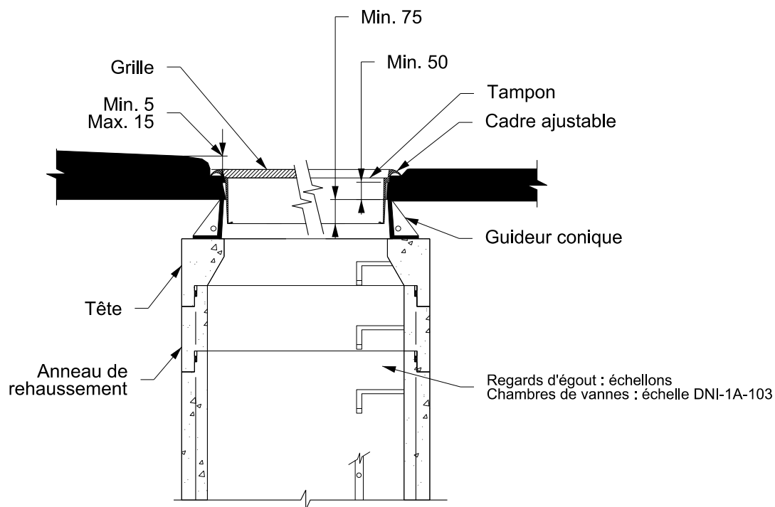
Ajustement des cadres dans les chaussées mixtes ou souples Coupe type
