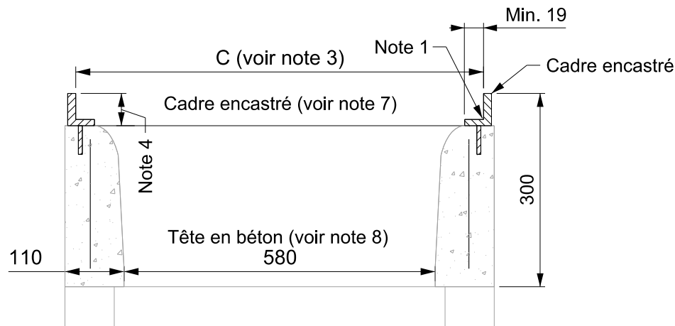
Tête en béton avec cadre encastré Coupe type
