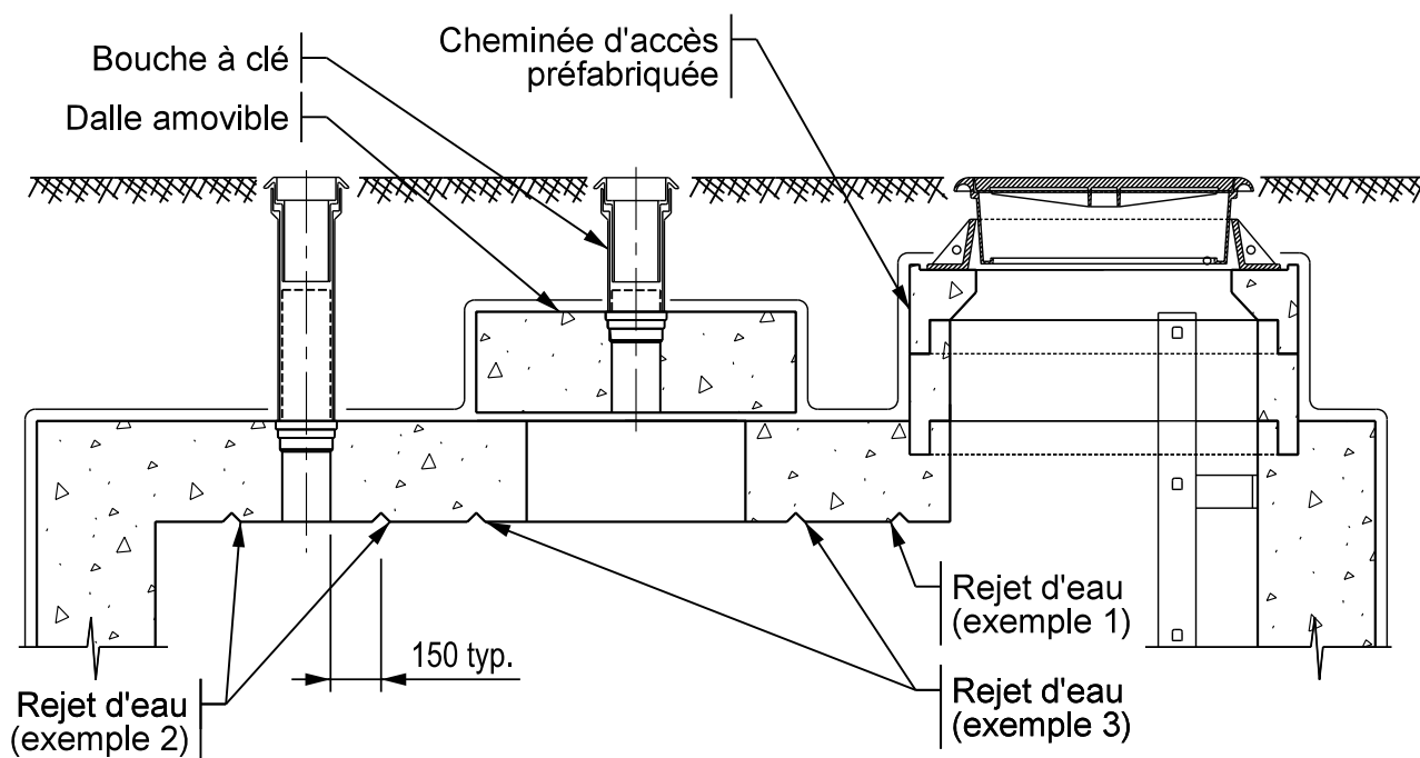
Vue en coupe
