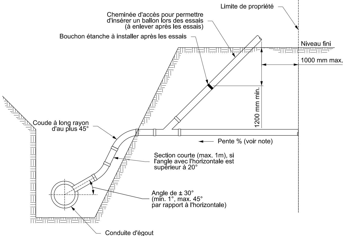
Élévation type
