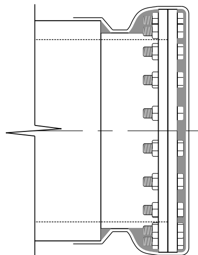
Trou d'accès enterré Voir notes
