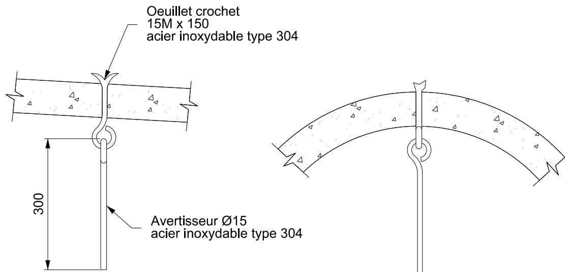
Détail
