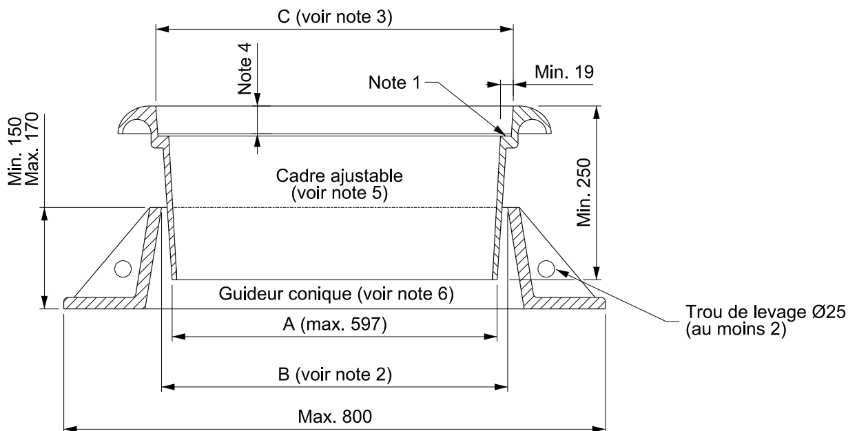
Type ajustable Coupe type
