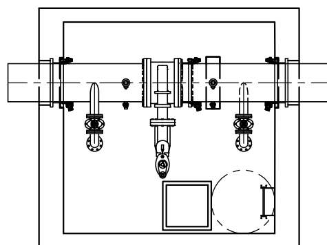
Vue en plan - Option #2
