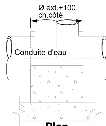
Plan Butée
