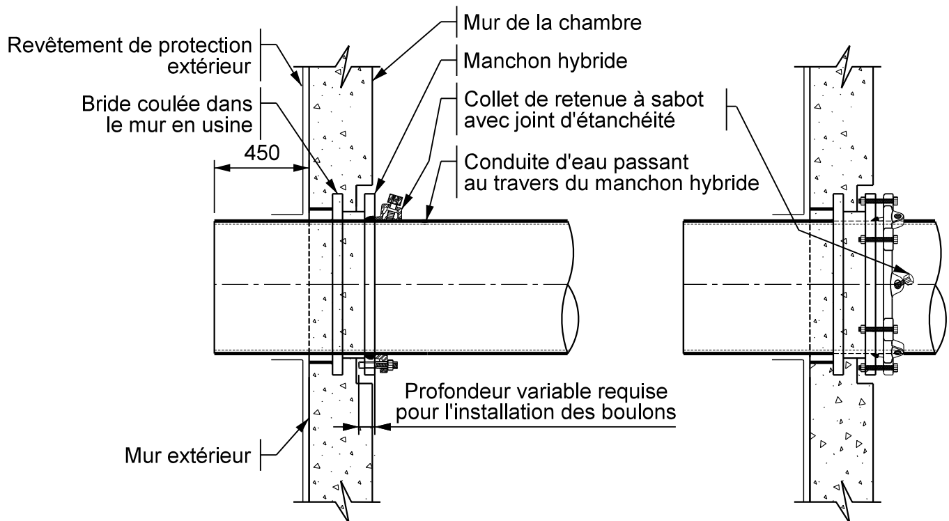
Système d'ancrage mural vue en coupe
