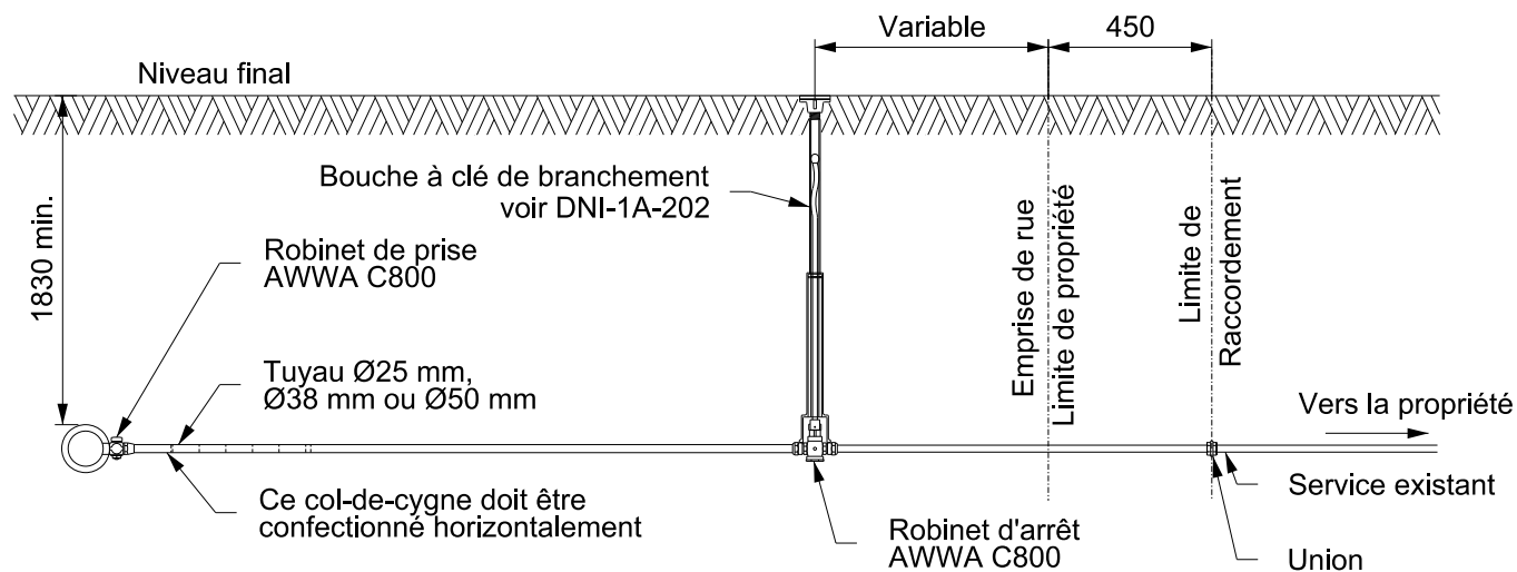
Élévation
