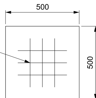
Dalle d'assise Vue en plan
