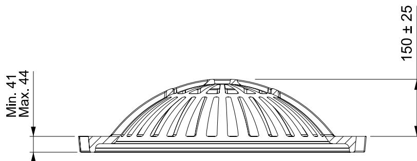
Grille en dôme pour puisard Coupe A-A
