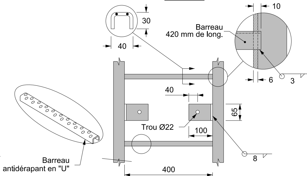
Détail B
