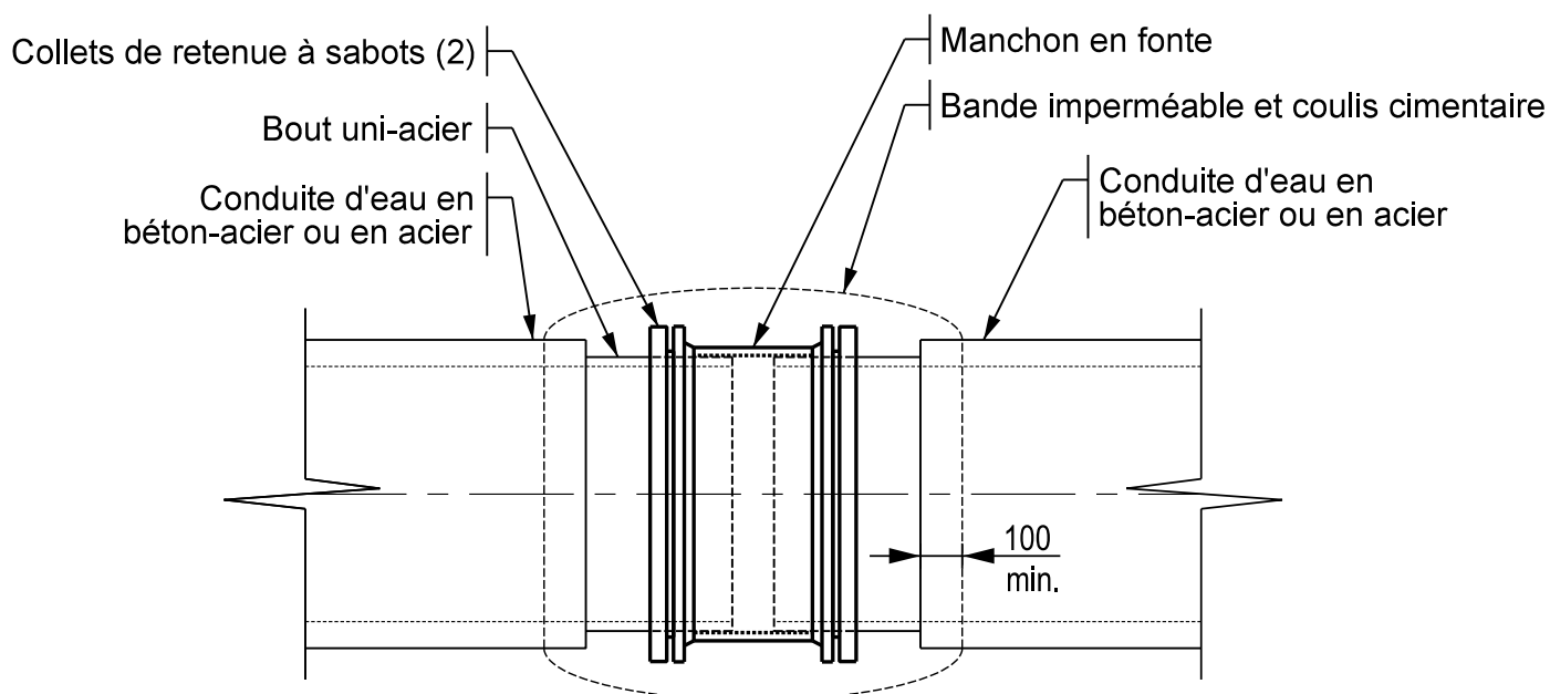
Raccord bout uni-acier à fonte
