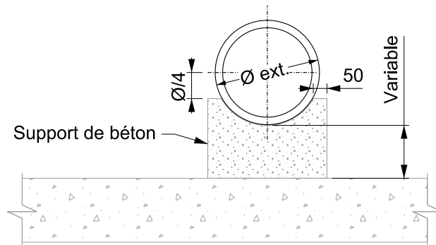
Coupe Conduite secondaire
