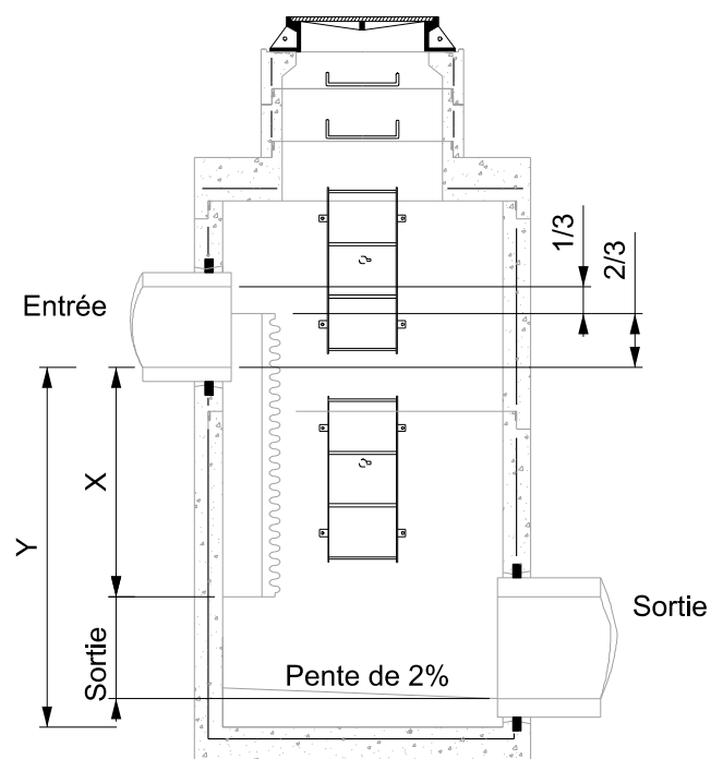
Coupe type
