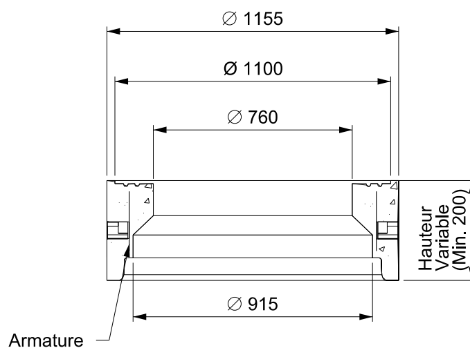
Tête Coupe type
