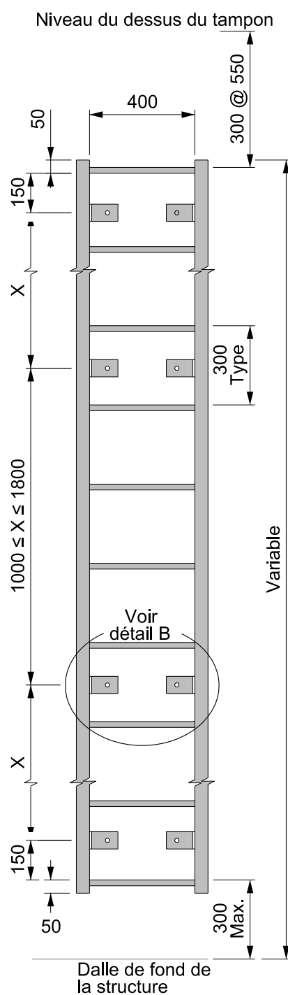
Élévation
