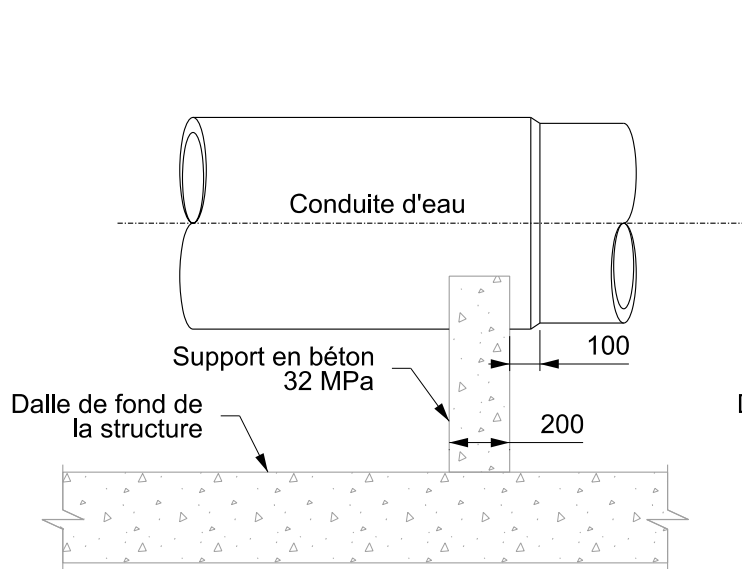
Profil Conduite principale
