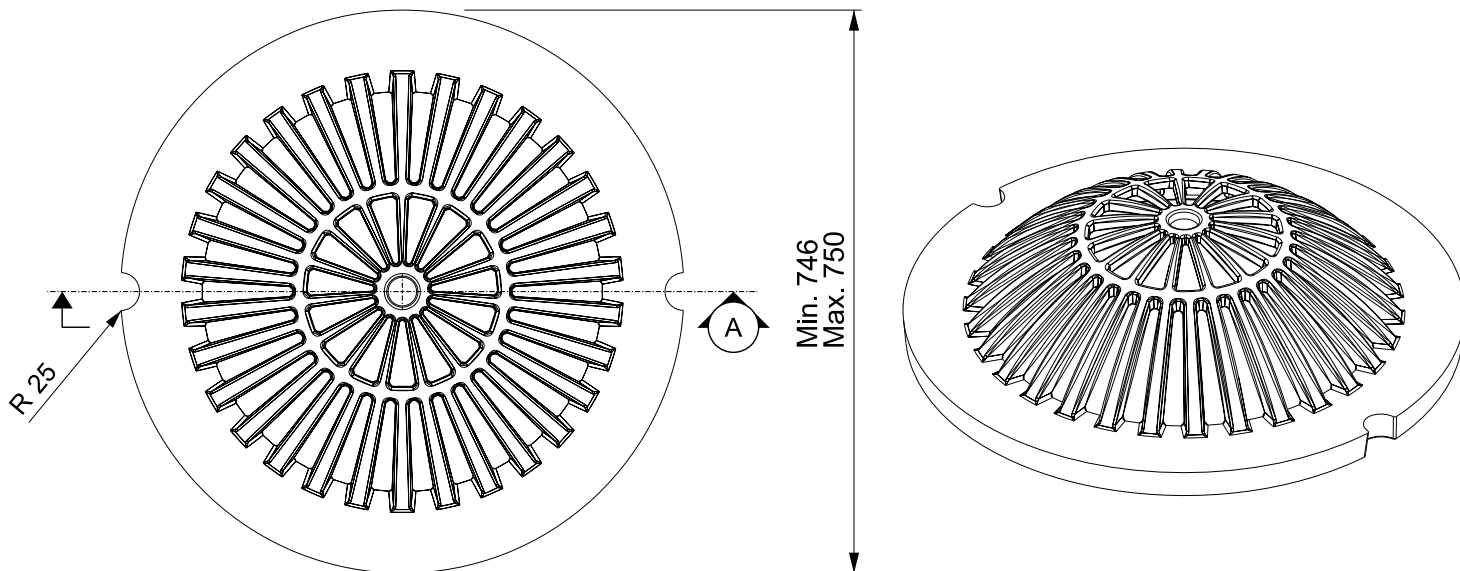
Grille en dôme pour puisard Vue en plan
