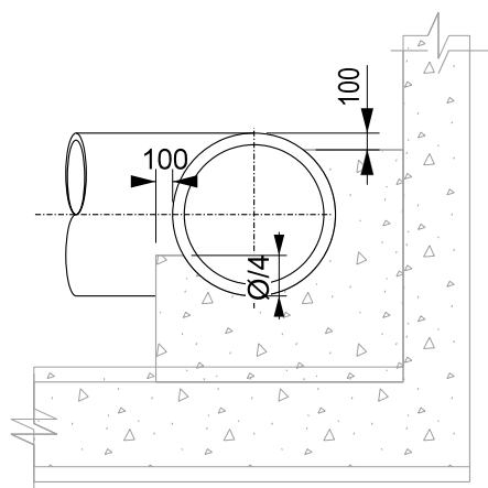
Coupe Butée
