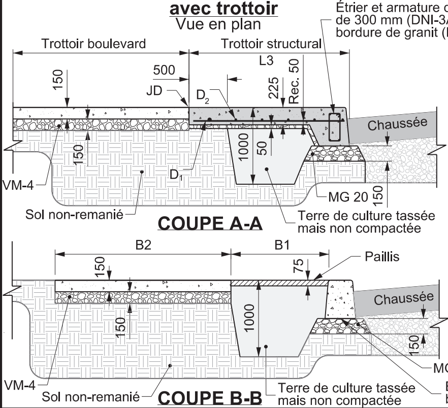
Fosses d'arbres combinées sans trottoir Vue en plan
