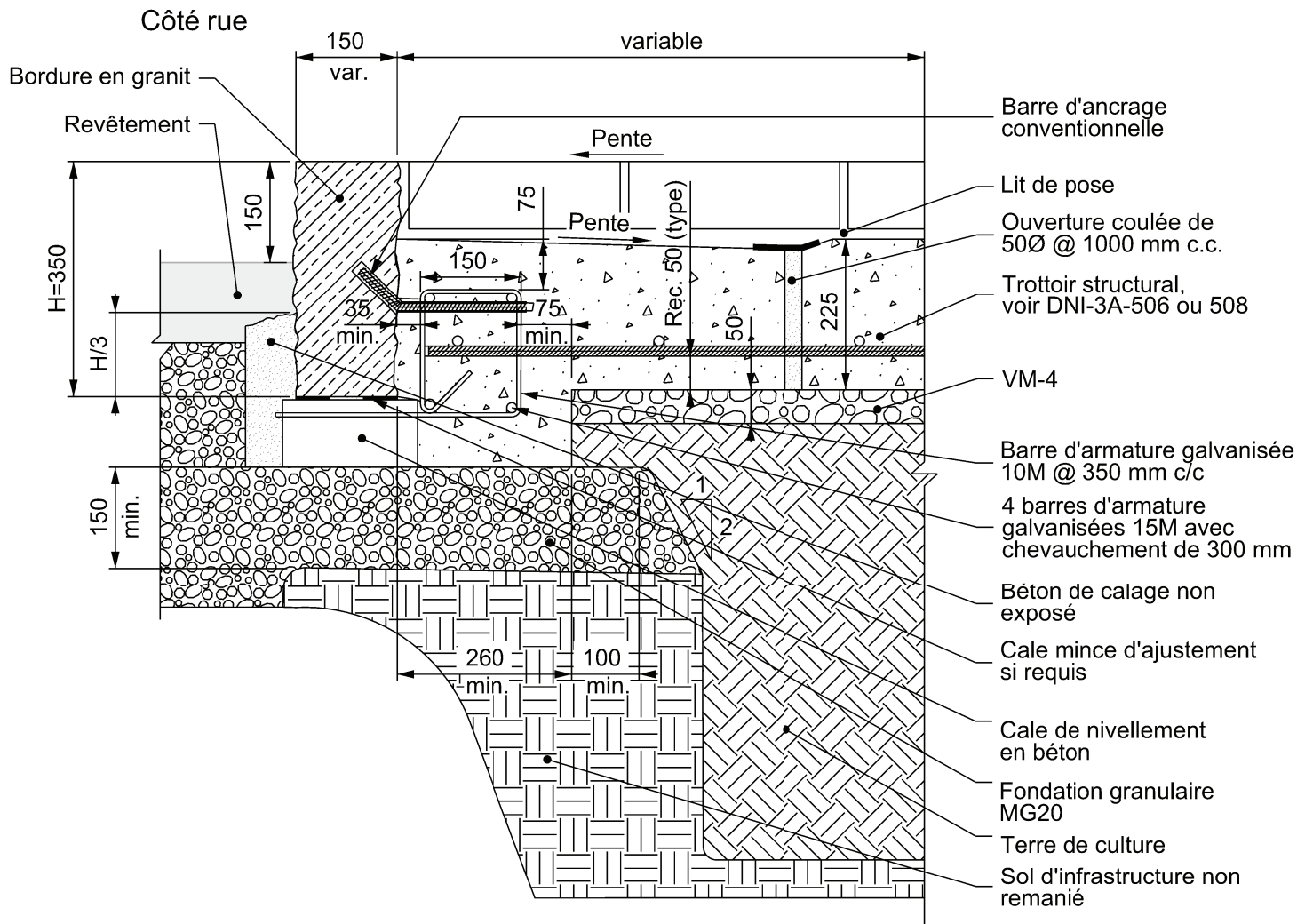
Coupe
