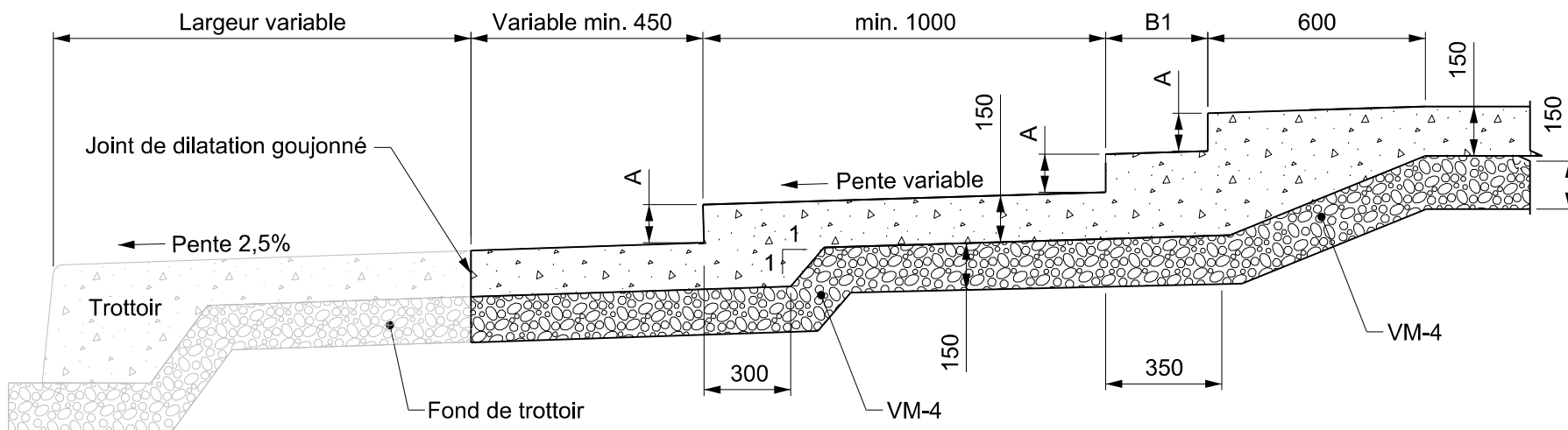
Élévation type
