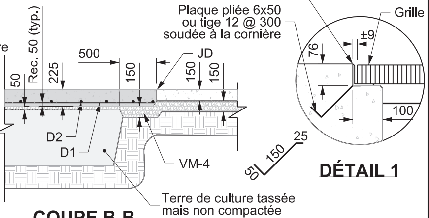
COUPE B-B
