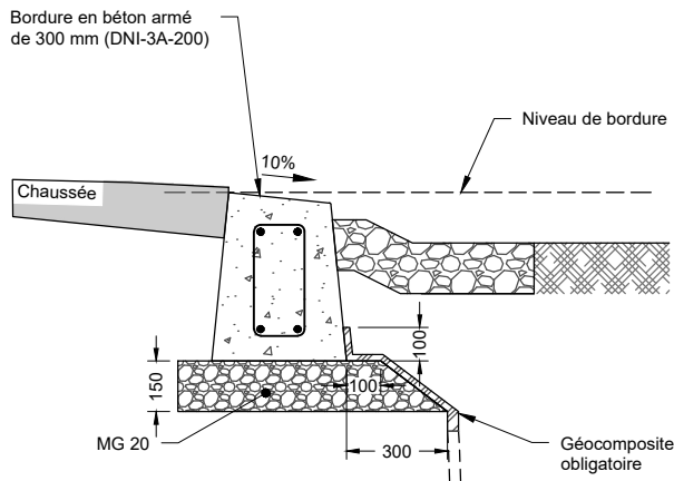
Bordure abaissée en béton armé Coupe
