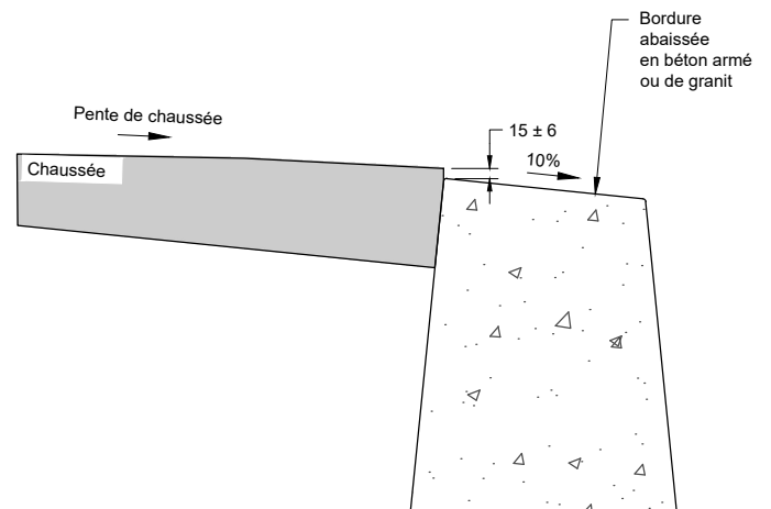
Niveau de bordure abaissée Coupe
