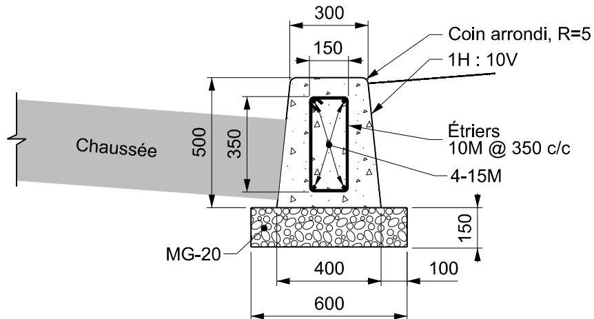
Bordure armée 300 mm
