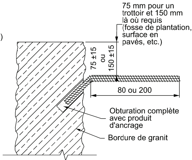
Installation de la barre d'ancrage
