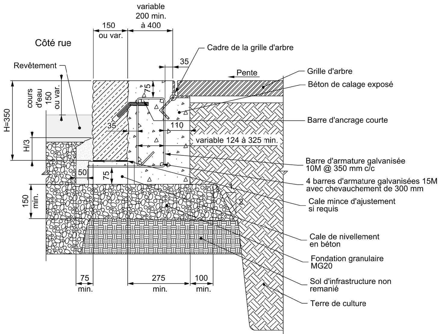
Coupe
