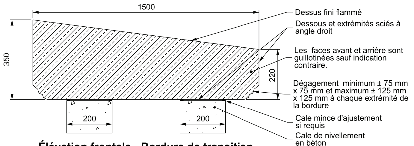
Élévation frontale - Bordure de transition
