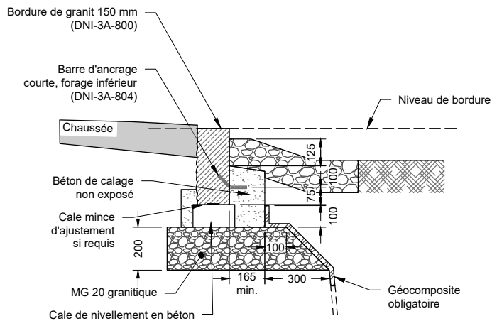
Bordure abaissée de granit Coupe
