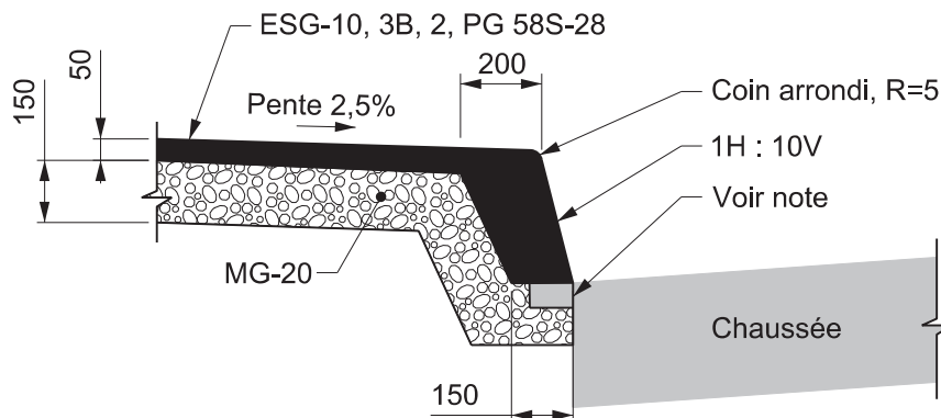
Trottoir et bordure temporaires Élévation type
