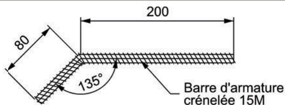
Barre d'ancrage conventionnelle
