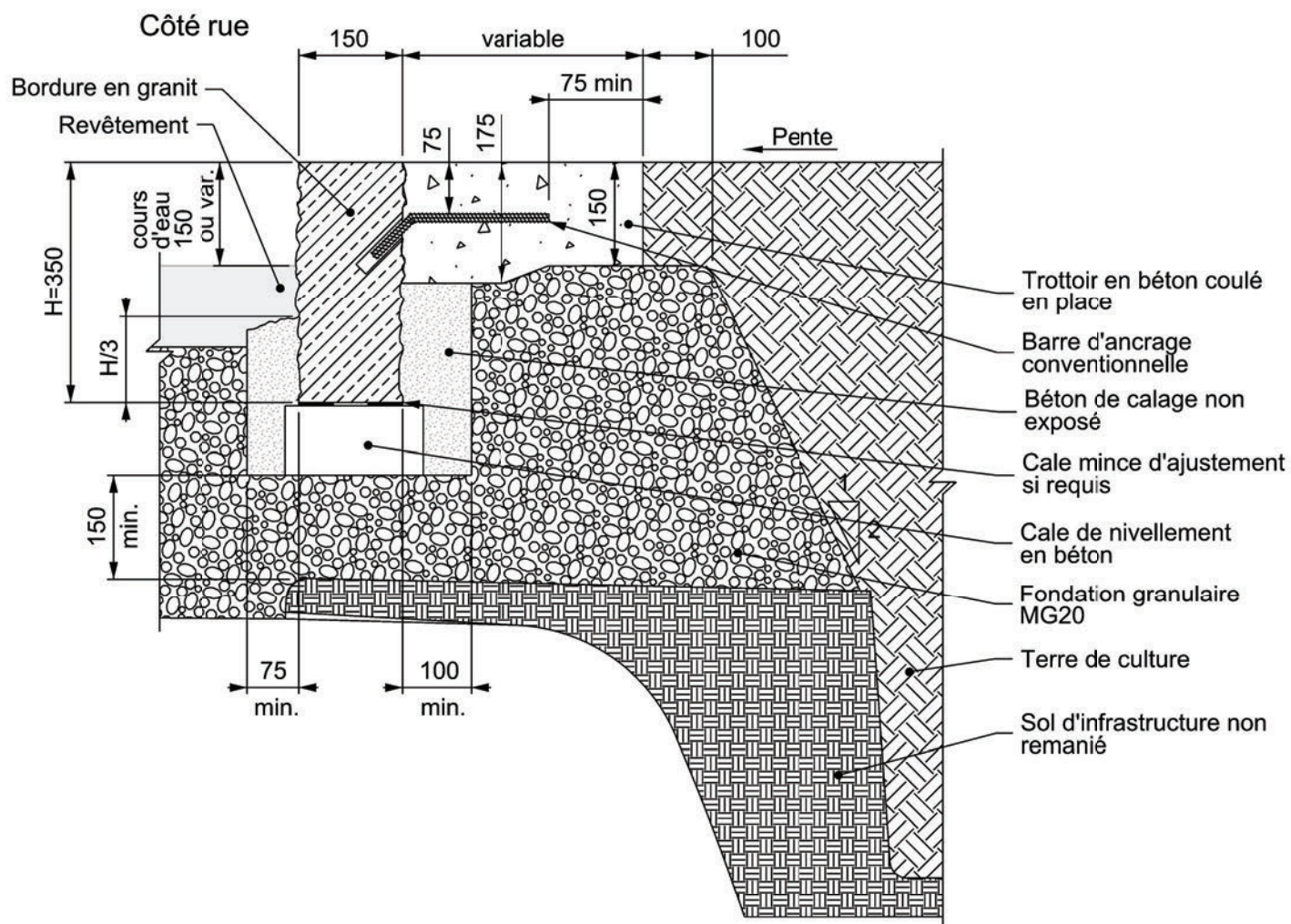
Coupe
