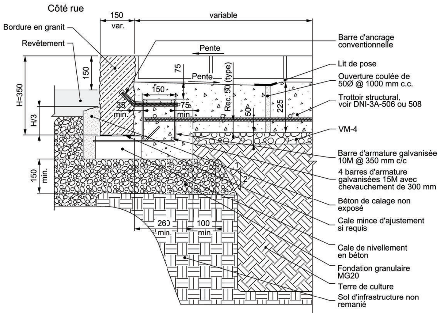
Coupe
