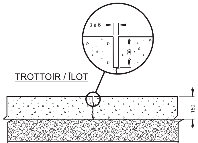
TROTTOIR SCIÉ ÉLEVATION TYPE
