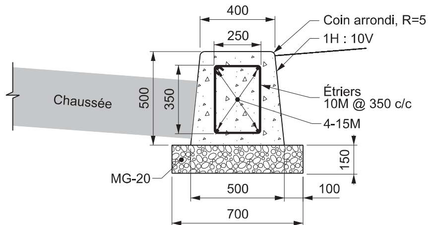
Bordure armée 400 mm
