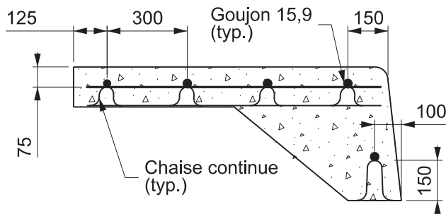
Trottoir monolithique
