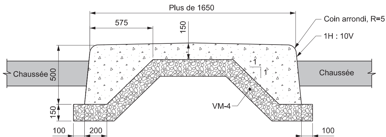
Élévation type
