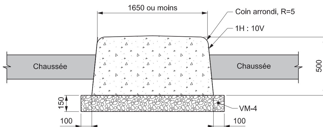
Élévation type
