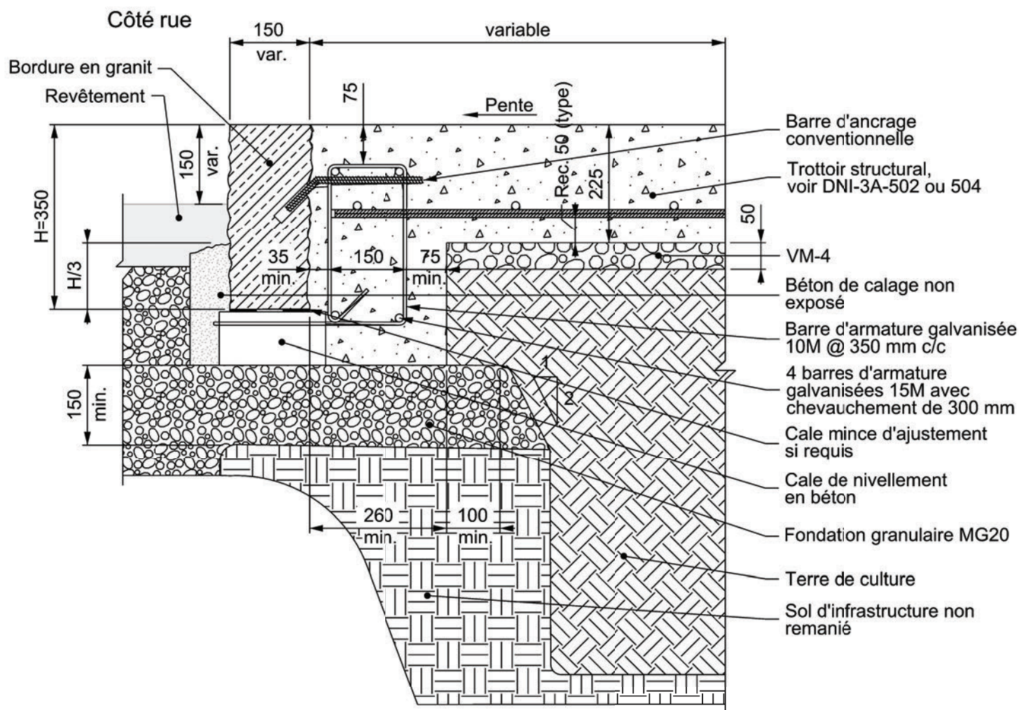
Coupe
