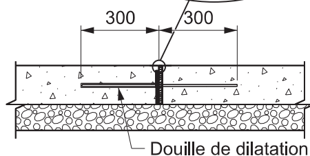
Joint de dilatation goujonné conventionnel
