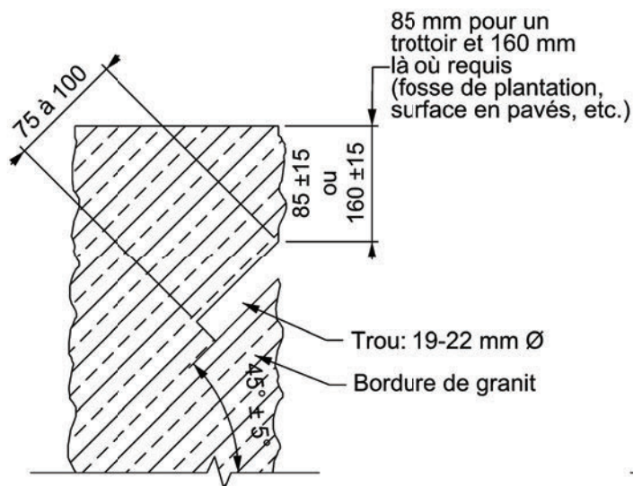
Forage supérieur
