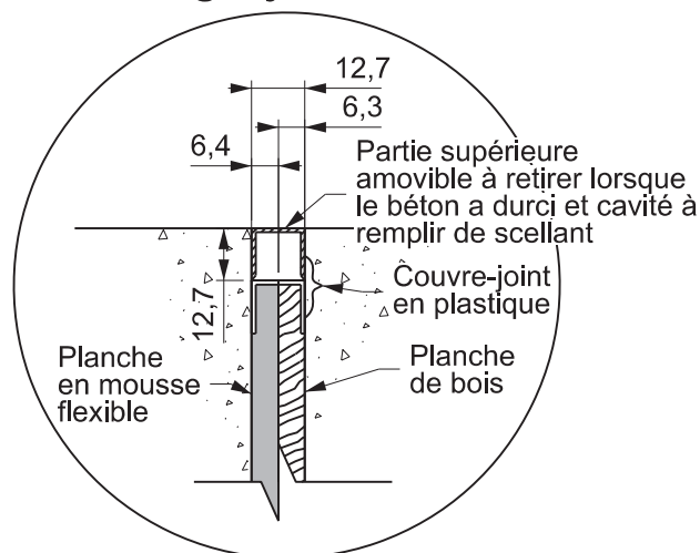
Joint de dilatation goujonné conventionnel
