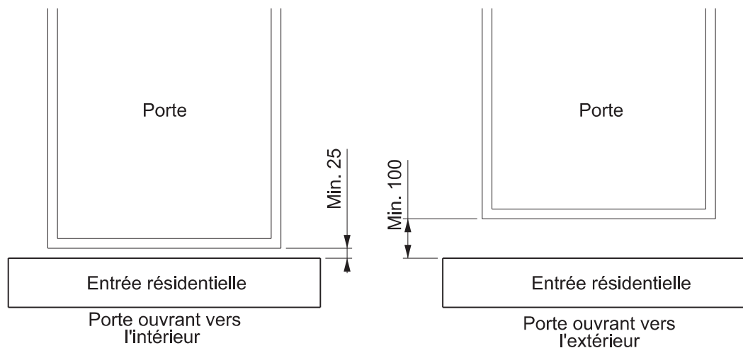
Élévation type
