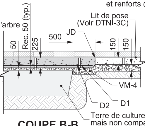
COUPE B-B
