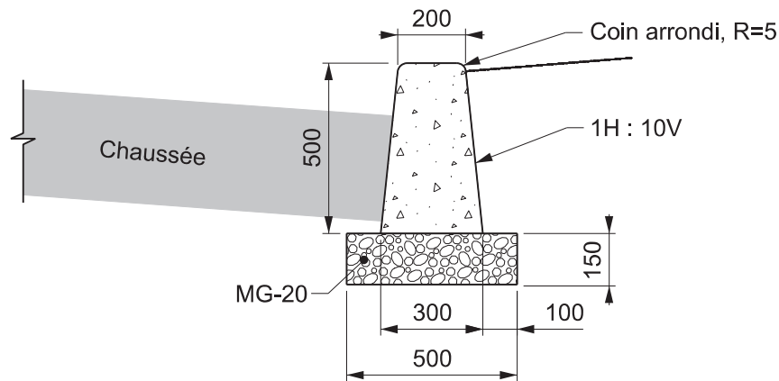
Bordure conventionnelle 200 mm
