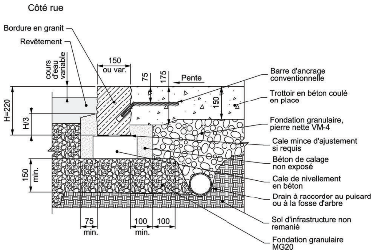
Coupe
