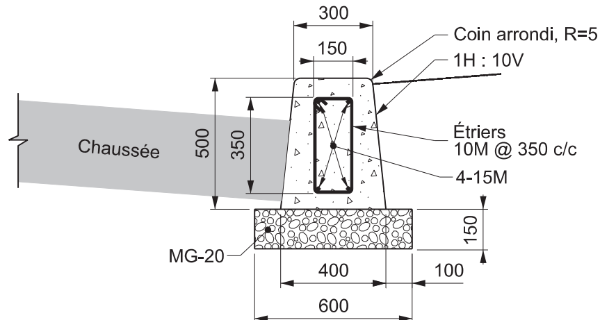
Bordure armée 300 mm
