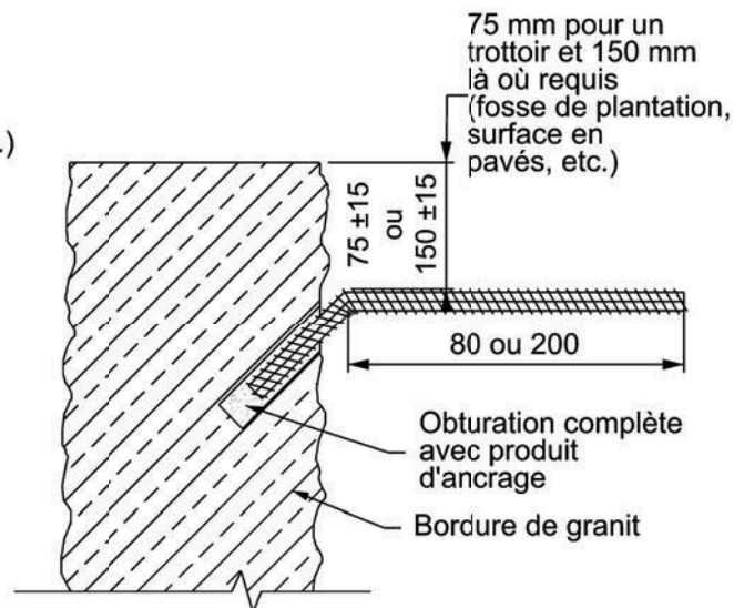
Installation de la barre d'ancrage
