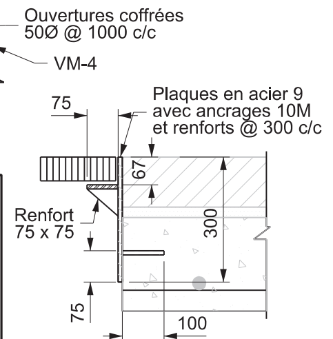
DÉTAIL 1
