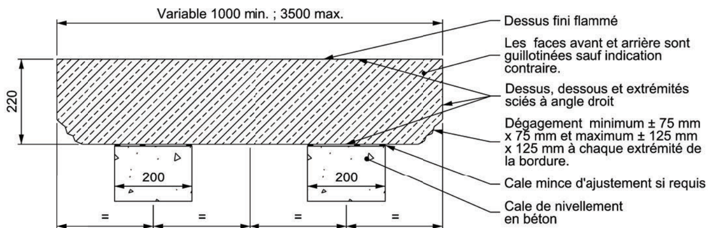
Élévation frontale
