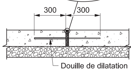
Joint de dilatation goujonné avec scellant
