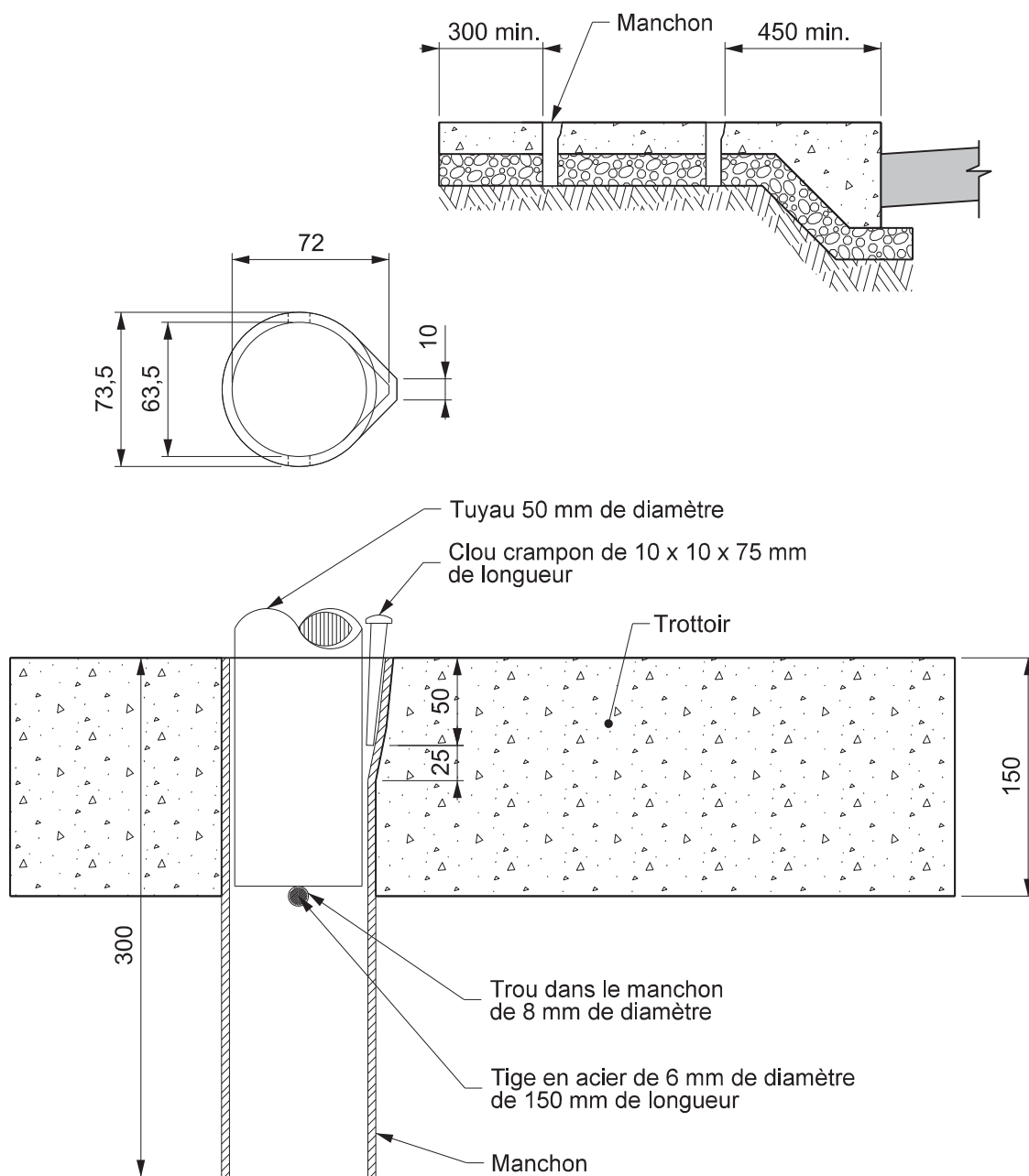
Élévation type
