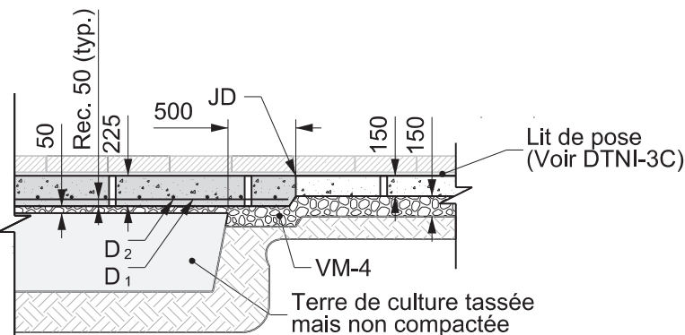
COUPE B-B
