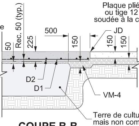
COUPE B-B
