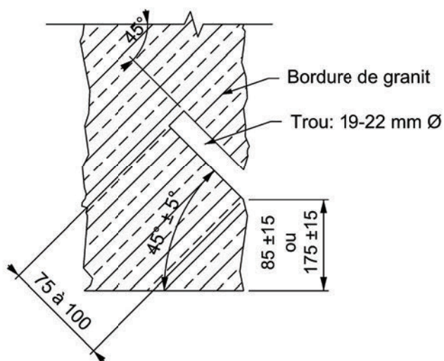
Forage inférieur
