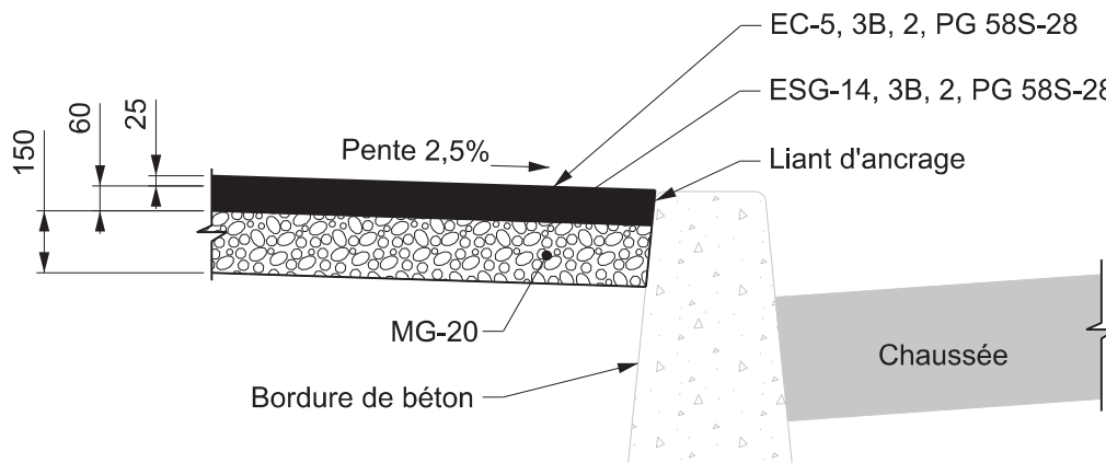
Trottoir permanent Élévation type
