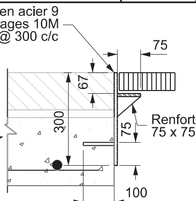
DÉTAIL 1
