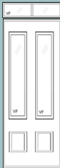
Porte simple Panneaux décoratifs en RELIEF Vitrage FIXE 2 sections 6,7 ou 8 po x 36 po (L x H) Imposte 1 ou 2 sections
