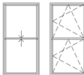
Fenêtre à guillotine \frac{1}{2} - \frac{1}{2} ;
