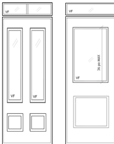
Porte simple Panneaux décoratifs en RELIEF (1 ou 2 sections) Vitrage FIXE 36 po ou 48 po maximum Imposte 1 ou 2 sections
