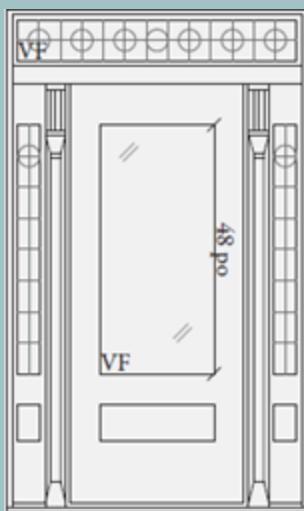
Porte simple avec impostes latéraux et vitraux Panneaux décoratifs en RELIEF Vitrage FIXE 48 po maximum et vitrail Pied-droit en bois de chaque côté de la porte Imposte avec vitraux
