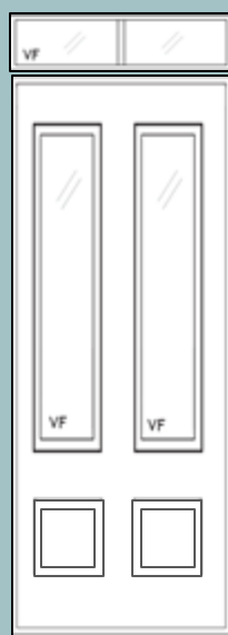
Porte simple Panneaux décoratifs en RELIEF Vitrage FIXE 2 sections 36 po ou 48 po Imposte 1 ou 2 sections
