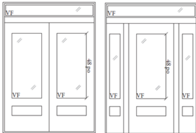
Porte double OU Porte simple avec impostes latéraux ET Panneaux décoratifs en RELIEF Vitrage FIXE 48 po maximum Imposte 1 section
