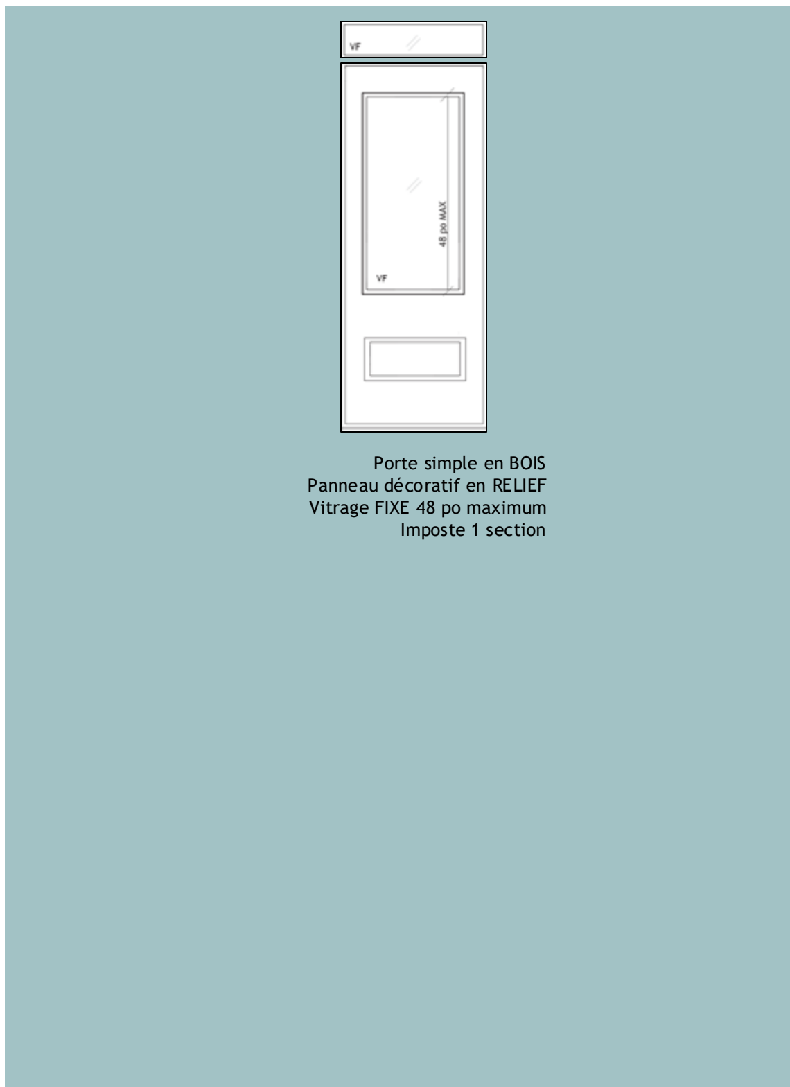
Porte simple EN BOIS
