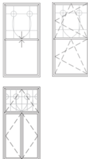
Fenêtre à crémonne 2 vantaux avec vitraux en contre-fenêtre
