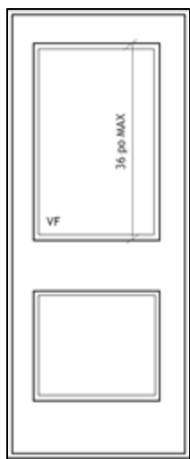
Porte simple Panneau décoratif en RELIEF Vitrage FIXE 20 ou 22 po x 36 po (LxH) Possibilité d'imposte
