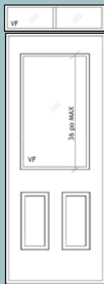
Porte simple Ornements, tablette ou panneaux décoratifs en RELIEF Vitrage FIXE 36 po maximum Imposte 1 ou 2 sections
