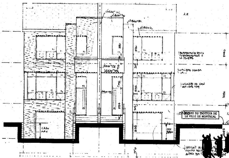
ELEVATION AVANT
