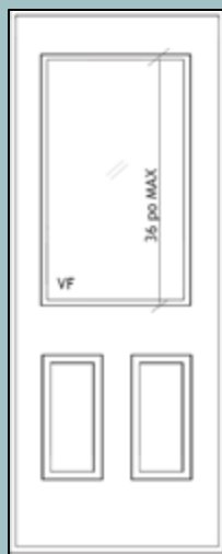
Porte simple Ornementations, tablette ou panneaux décoratifs en RELIEF Vitrage FIXE 36 po maximum Imposte 1 ou 2 sections
