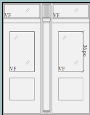
Porte simple, jumelée Panneaux décoratifs en RELIEF Vitrage FIXE 48 po maximum Pied-droit en bois au centre Impostes
