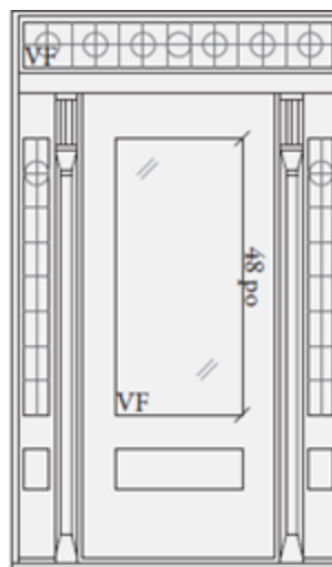
Porte double OU Porte simple avec impostes latéraux ET Panneaux décoratifs en RELIEF Vitrage FIXE 48 po maximum Imposte 1 section
