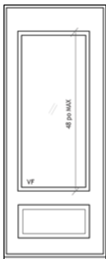
Porte simple Panneau décoratif en RELIEF Vitrage FIXE 20 ou 22 po x 48 po (LxH) Possibilité d'imposte
