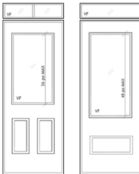
Porte simple Panneaux décoratifs en RELIEF (1 ou 2 sections) Vitrage FIXE 36 po ou 48 po maximum Imposte 1 ou 2 sections
