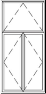
Fenêtre à guillotine \frac{1}{3} - \frac{2}{3} avec battants intérieurs (crémone) ou coulissant
