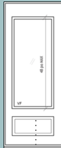
Porte simple Composition 1, 2 ou 3 rangées Panneaux décoratifs en RELIEF 1 ou 2 sections Vitrage FIXE 50 % maximum
