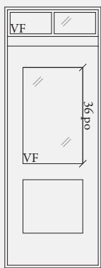
Porte simple avec imposte vitrage 20 po ou 22 po X 36 po
