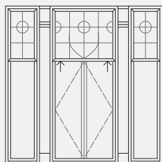
Fenêtres à guillotine 1/3-2/3 avec battants intérieurs, fenêtres latérales fixes et pieds-droits
