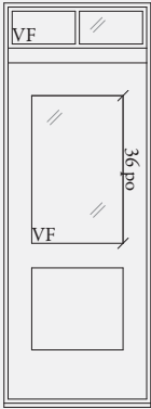
Porte simple avec imposte vitrage 20 po ou 22 po X 36 po
