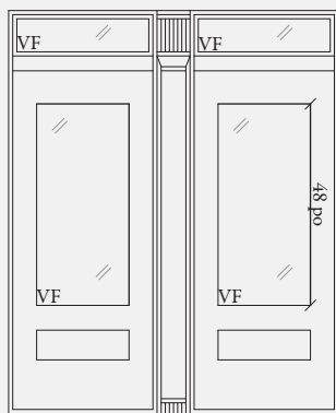
Portes simples avec imposte, jumelées vitrage 20 po ou 22 po X 48 po pied-droit séparant les portes
