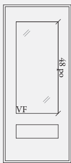
Porte simple vitrage 20 po ou 22 po X 48 po
