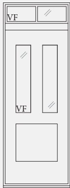
Porte simple avec imposte vitrage divisé en deux sections verticales
