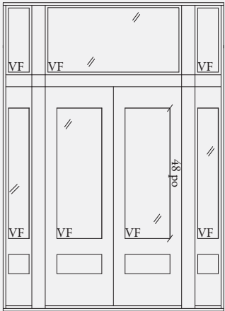
Portes doubles avec fenêtres latérales fixes et imposte vitrage 20 po ou 22 po x 48 po
