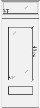
Porte simple avec imposte vitrage 20 po ou 22 po X 48 po
