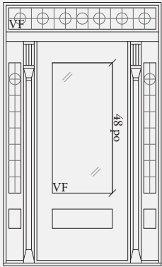
Porte simple avec fenêtres latérales fixes et imposte vitrage 20 po ou 22 po x 48 po
