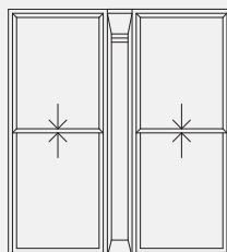
Fenêtres à guillotine 1/2-1/2 avec pied-droit
