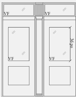
Portes simples avec imposte, jumelées vitrage 20 po ou 22 po X 36 po pied-droit séparant les portes
