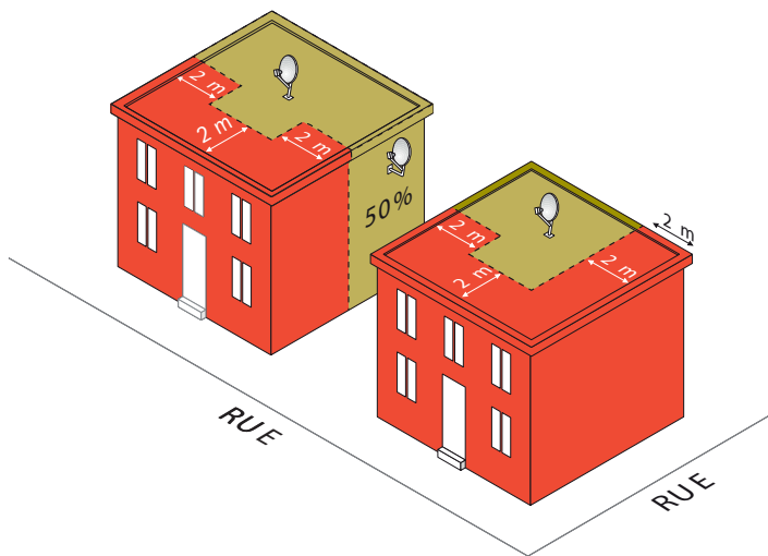
Illustration 3 : Emplacement d'une antenne satellite sur un toit plat
