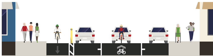
Coupe de la rue entre le boulevard Saint-Laurent et la rue Saint-Denis (vue vers l'ouest)
