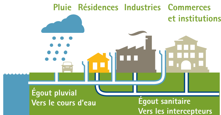
Réseau séparatif
